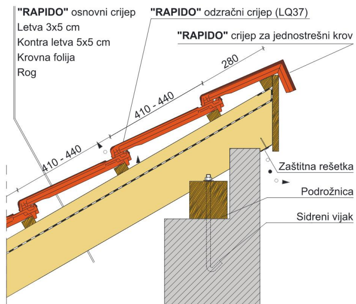
Jednostresni krov
